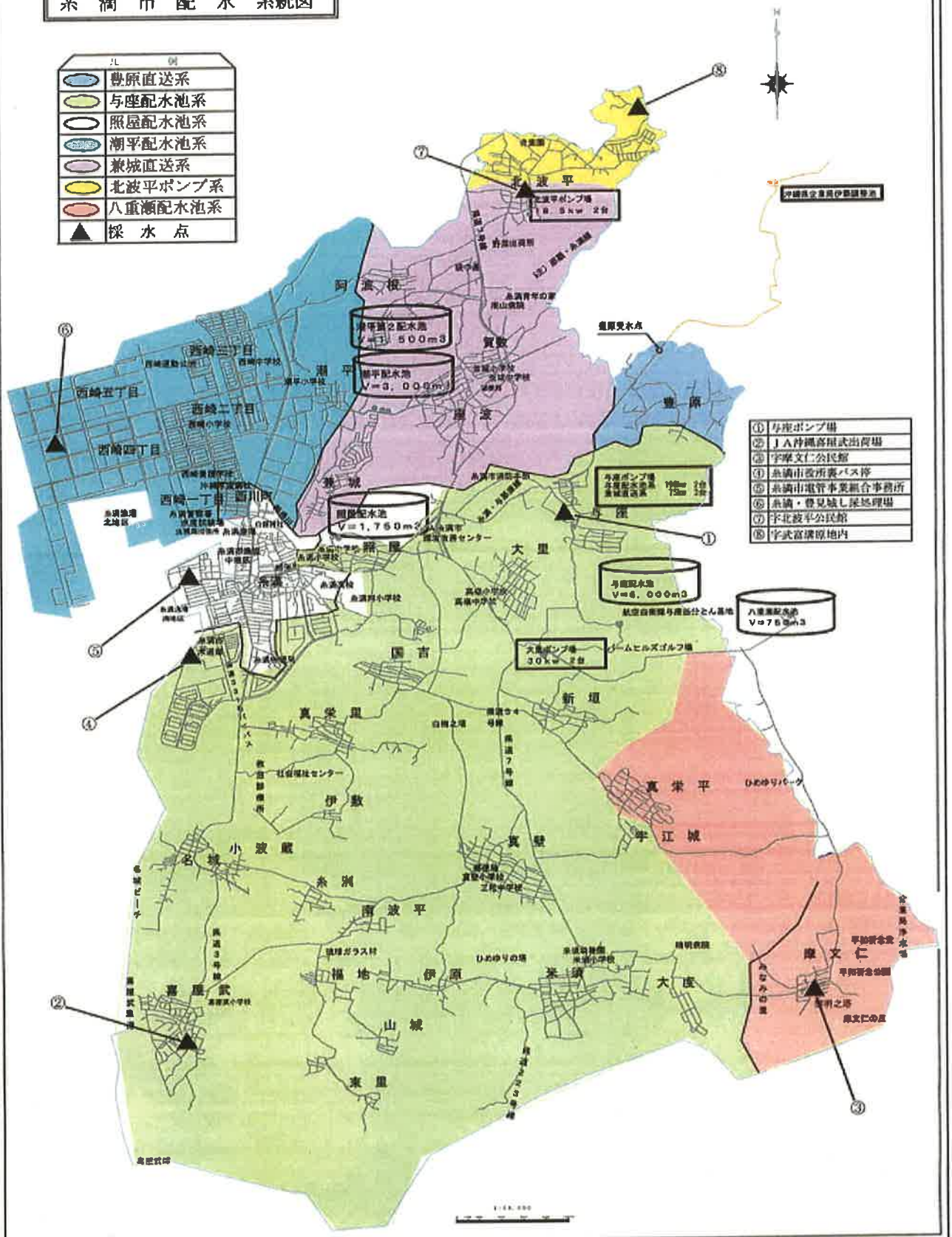
糸満市配水系統図
