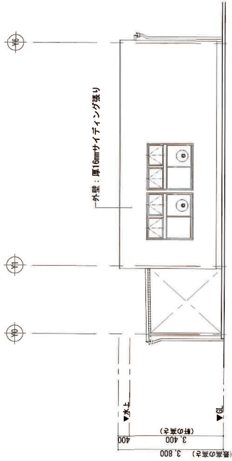
東側立面図 S=1/100
